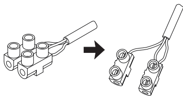
Рисунок 4 — Разделение секций клеммной колодки
