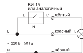
Рисунок 3 — Схема подключения светильника СА-7106Е к питающей сети при использовании внешнего датчика ВИ-15
