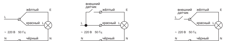
а) Схема подключения без использования внешнего датчика
